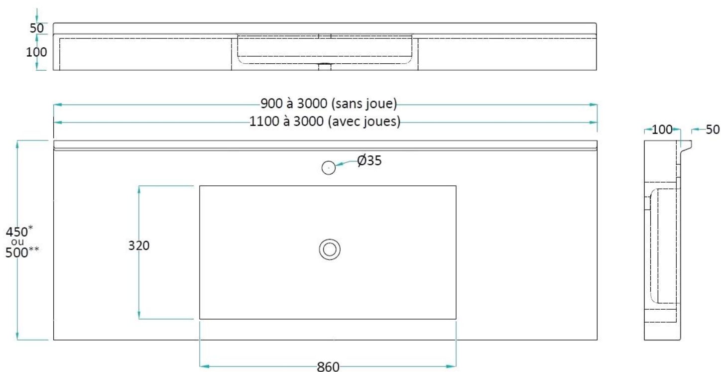
Version Surian Platine S7036, sans trop plein
