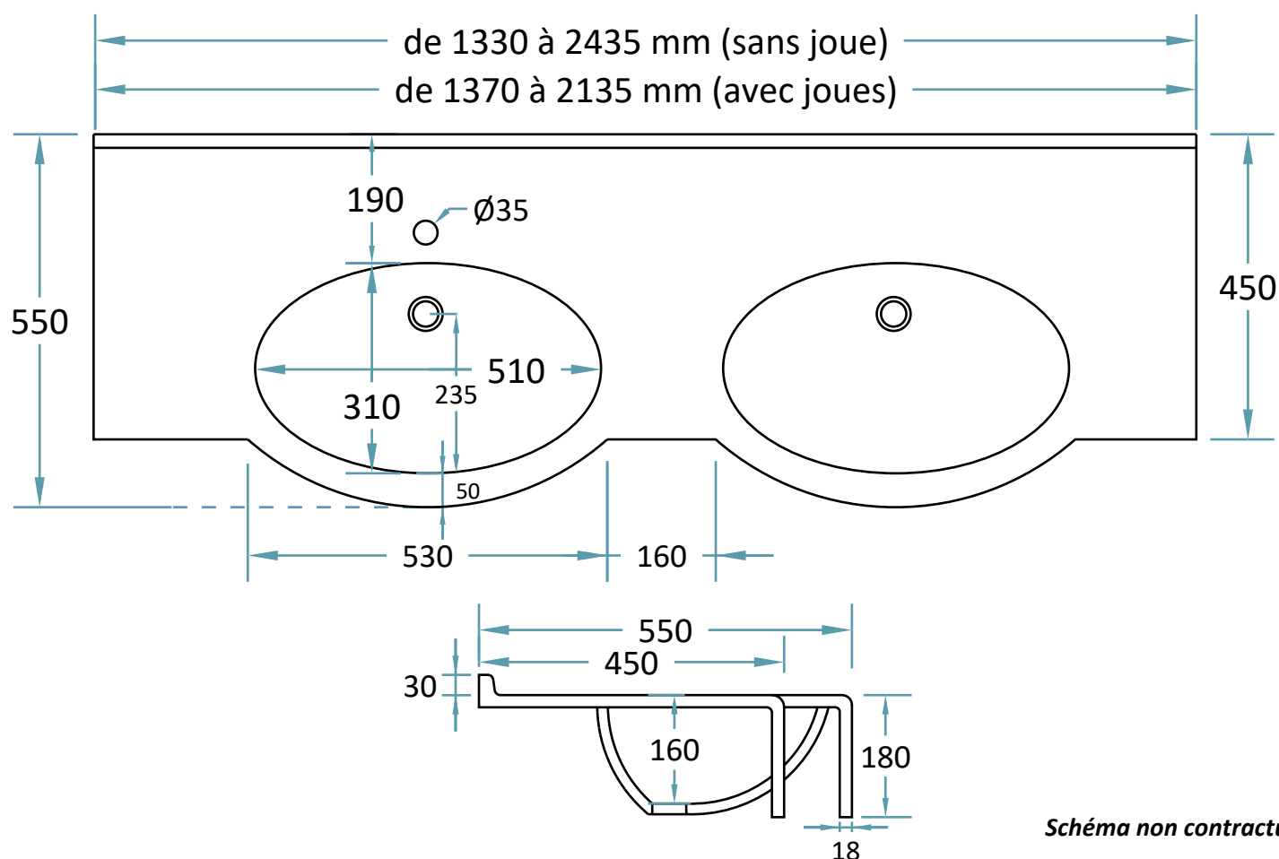
Version Marbol Blanc, sans trop-plein
