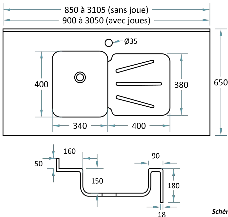
Version Surian Blanc S250, avec trop-plein et perçage en façade
