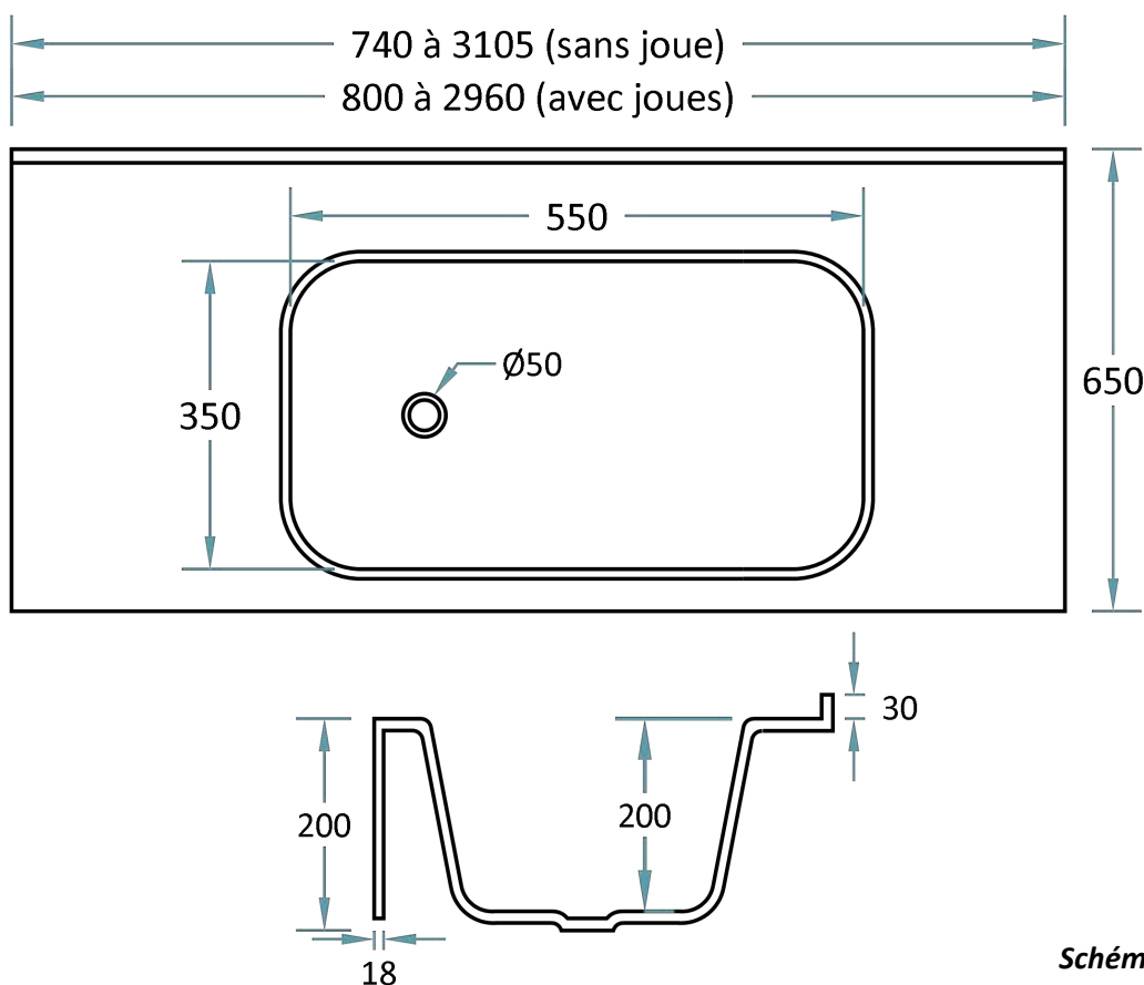
Version Surian Blanc S250, avec trop-plein et dossierets latéraux rapportés
